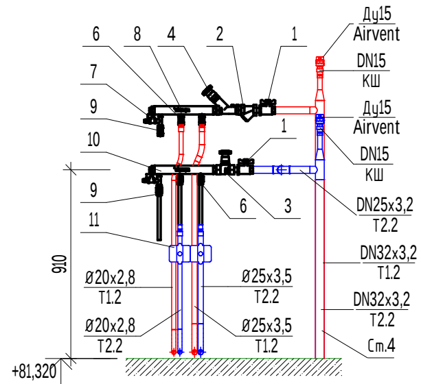
Коллектор на 2 выхода (28 этаж, Ст.4)
